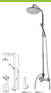
RAMPA CHUV.NAO TELESCOPICA C/MNC. ZOLA GO CR Ref.ª WZOLA005GOAQ
